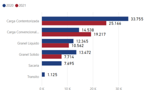
Mês de Março - Porto da Praia: Mov. Mercadorias (ton) por Tipo de Carga
